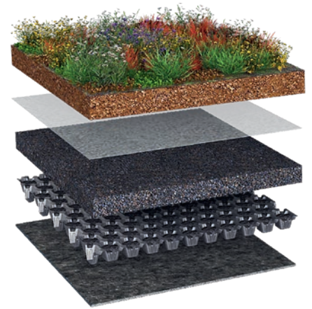
Dieser Retentionsdachaufbau aus der Serie BauderGREEN sorgt für eine besonders starke Verdunstung.
